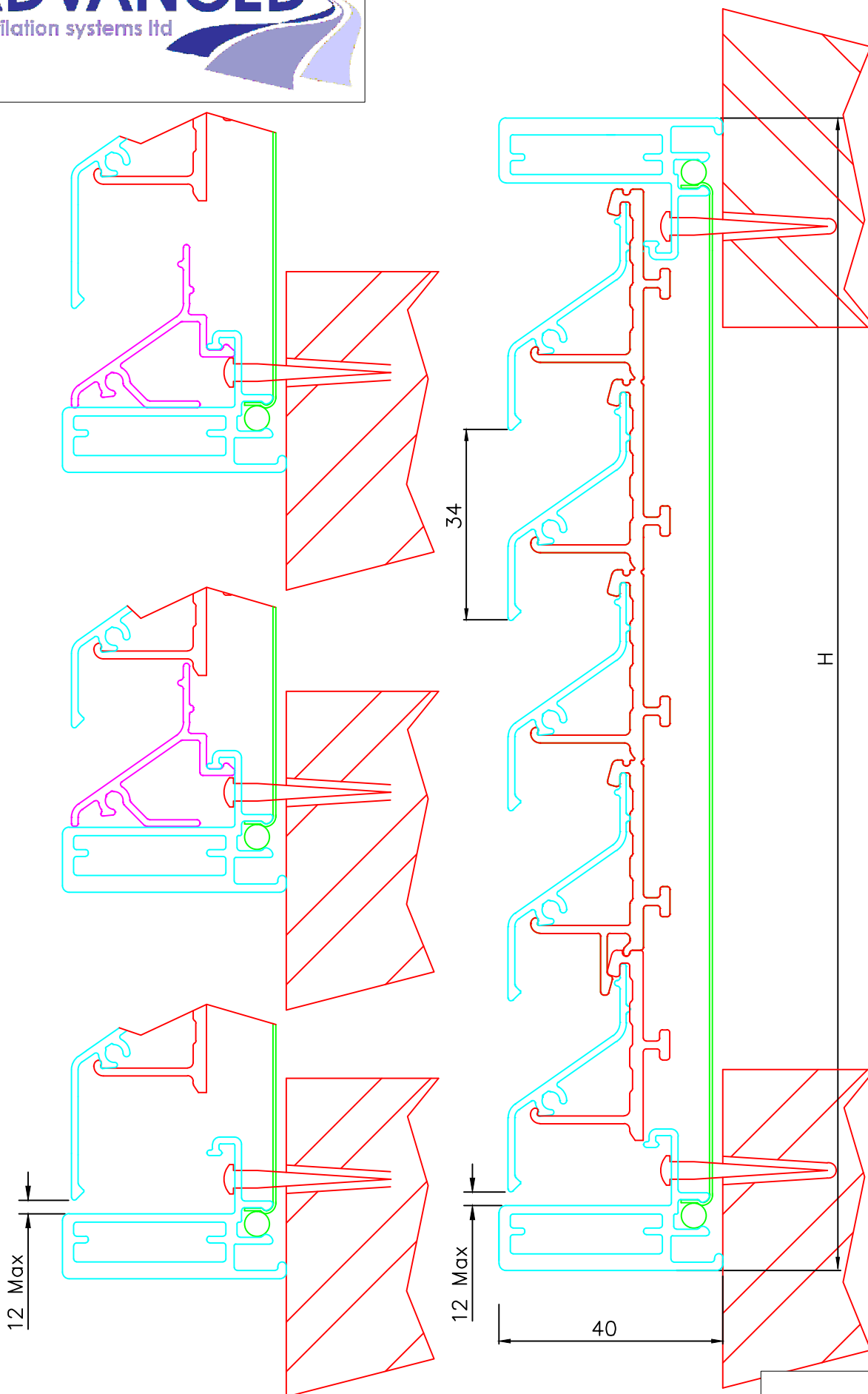
AVS34SM Vertical Section 1:1
