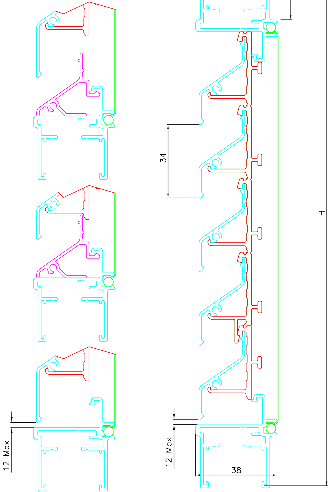
AVS34GL32 Vertical Section 1:1
